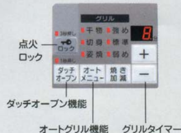
●グリル操作パネル
